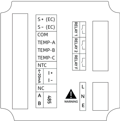
220V 一路 4~20mA 接线图
