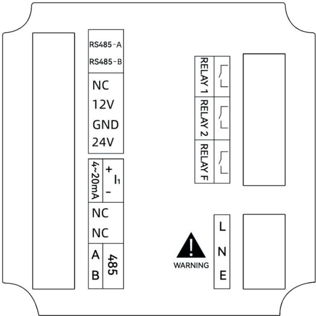
220V 接线图
